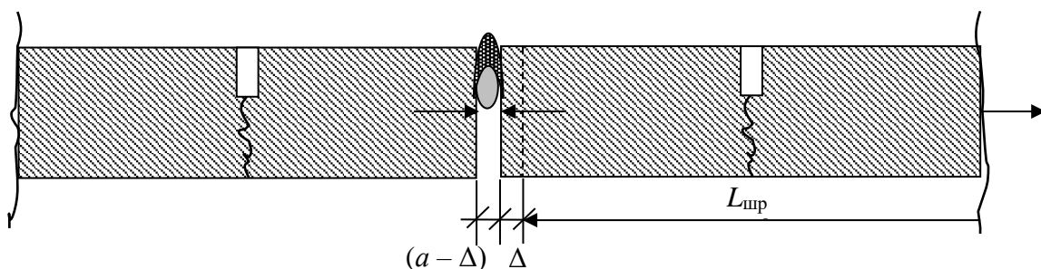
б) Обжатие прокладки (герметика) в шве при расширении бетона
