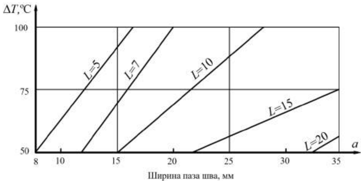
Рисунок 8.4 – Номограмма для определения ширины паза шва при использовании герметизирующего материала с относительным удлинением \varepsilon = 50\% при температуре минус 20\text{ °C}
