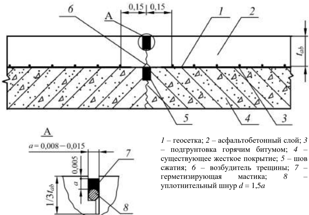
Рисунок 9.5 – Деформационный шов в однослойном асфальтобетонном покрытии
