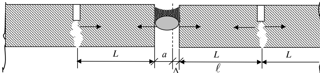
в) Растяжение герметика в шве при сжатии бетонной плиты длиной L
