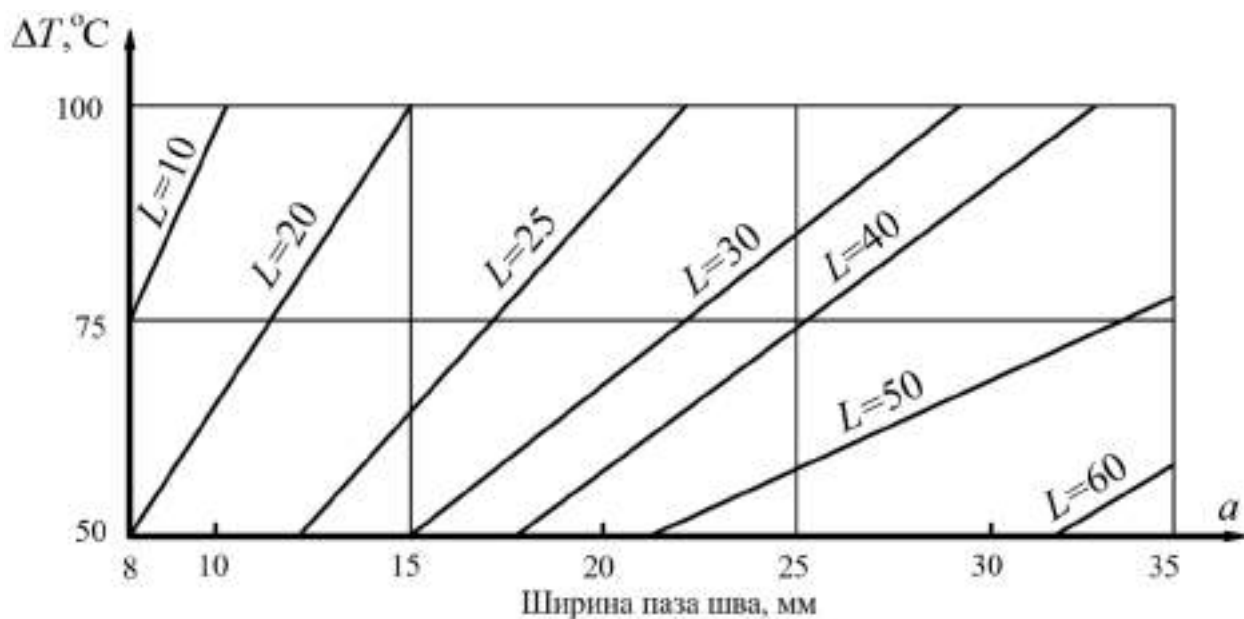
Рисунок 8.6 – Номограмма для определения ширины паза шва при использовании герметизирующего материала с относительным удлинением \varepsilon = 150\% при температуре минус 20\text{ }^{\circ}\text{C}
