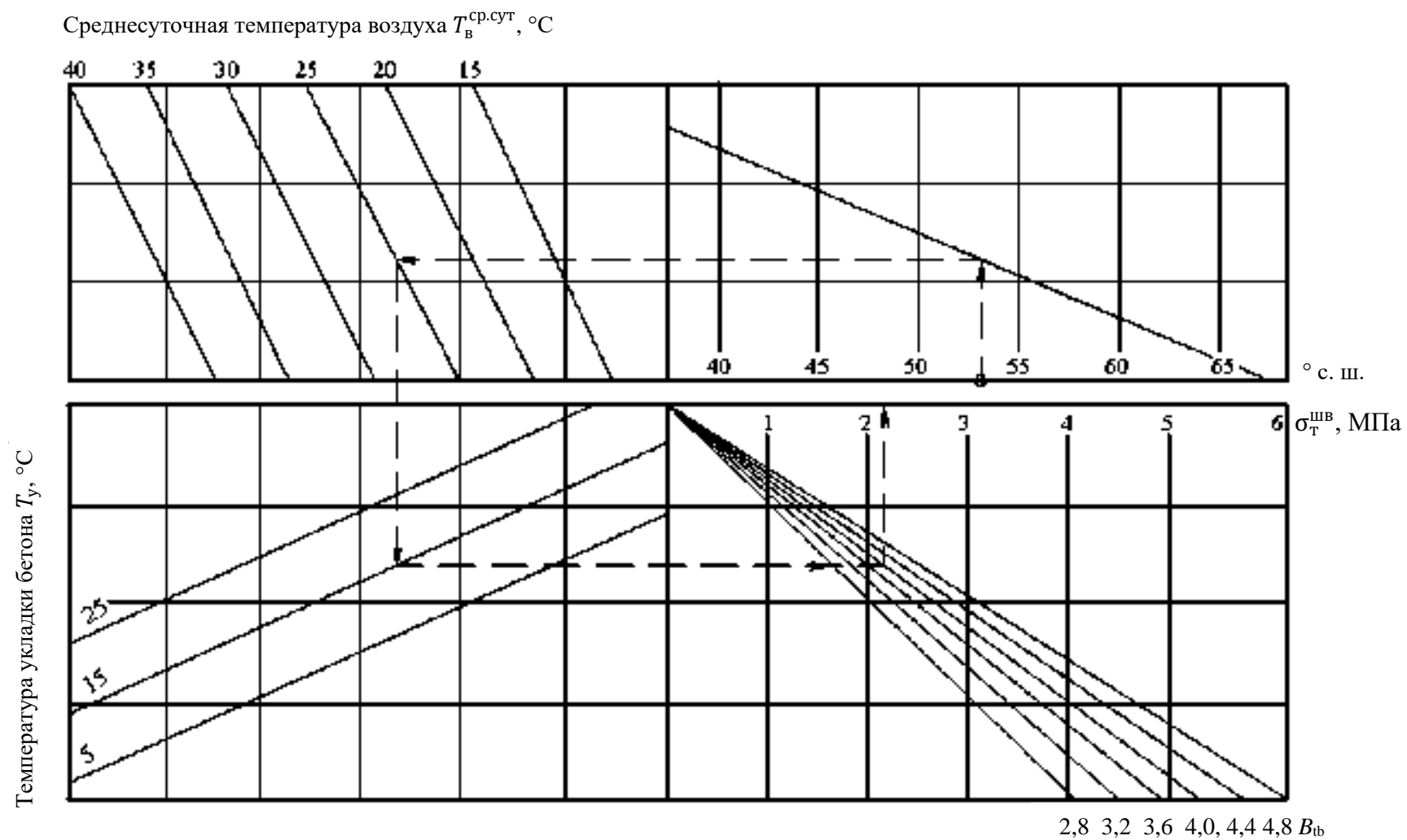
Рисунок 13.1 – Номограмма для определения температурных напряжений \sigma_{\text{т}}^{\text{шв}} на краю плиты
