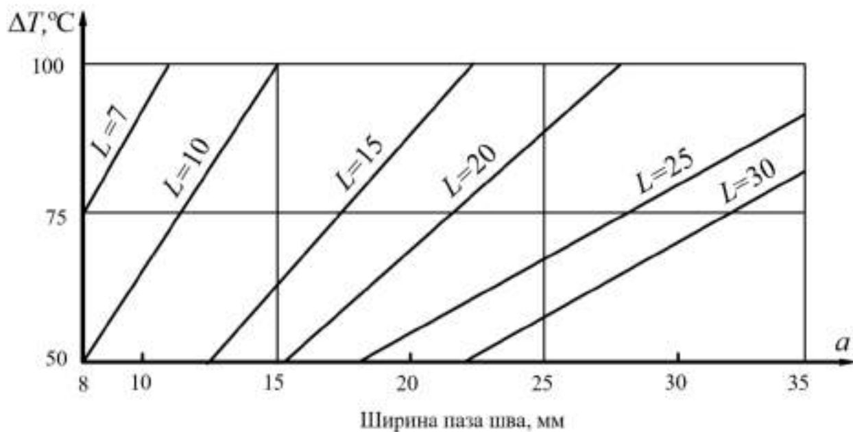
Рисунок 8.5 – Номограмма для определения ширины паза шва при использовании герметизирующего материала с относительным удлинением \varepsilon = 100\% при температуре минус 20\text{ °C}
