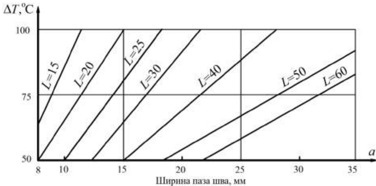
Рисунок 8.7 – Номограмма для определения ширины паза шва при использовании герметизирующего материала с относительным удлинением \varepsilon = 200\% при температуре минус 20\text{ }^{\circ}\text{C}
