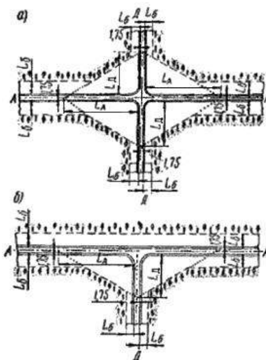
Рисунок 6.2 - Схемы обеспечения видимости
