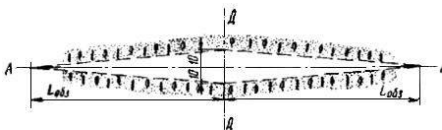
Рисунок 6.3 - Схема видимости по главной дороге и обзорности с второстепенной дорогой
