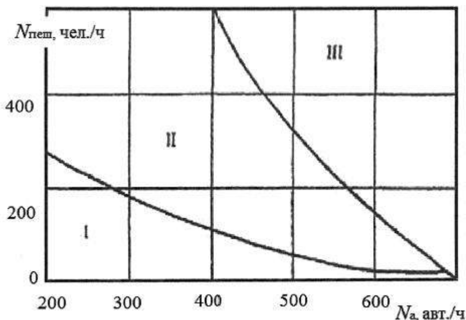
Рисунок 6.1 - Области применения пешеходных переходов различных типов
